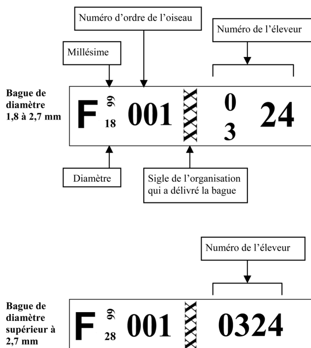
Schéma du déroulé des bagues fermées
